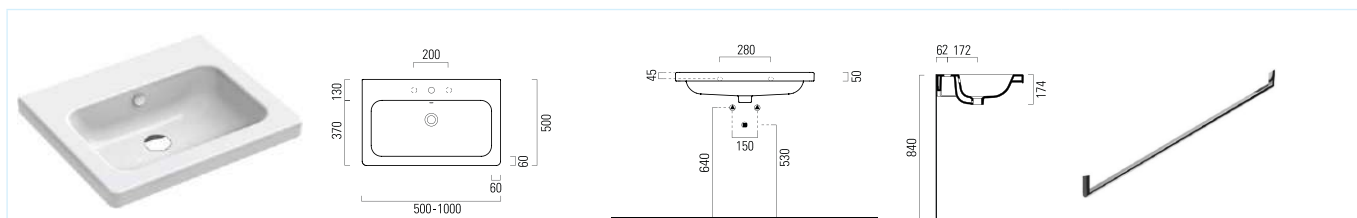
Umyvadlo s úpravou concept - clean PLUS bez otvoru s přep., 60 × 50 cm (kód 60CO200EXCBOH) bez otvoru s přep., 65 × 50 cm (kód 65CO200EXCBOH) bez otvoru s přep., 80 × 50 cm (kód 80CO200EXCBOH) bez otvoru s přep., 100 × 50 cm (kód 100CO200EXCBOH)
