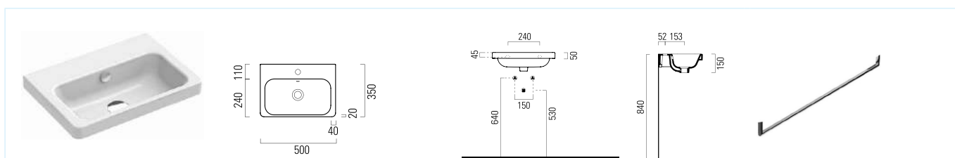
Umyvadlo s úpravou Concept - clean PLUS bez otvoru s přepadem, 50 × 35 cm (kód 50CO200EXCBOH) s otvorem a přepadem, 50 × 35 cm (kód 50CO200EXCB)
