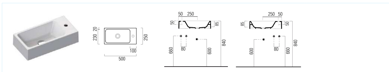
Umyvátko s úpravou Concept - clean PLUS s otvorem a přepadem, 50 × 25 cm (kód 5025CO200EXCB)
